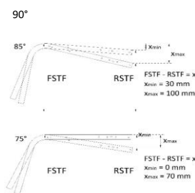
Pente d'assise en fonction du type de châssis
